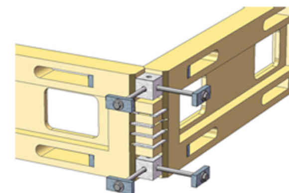
Holzbausystem Cross House, CH
